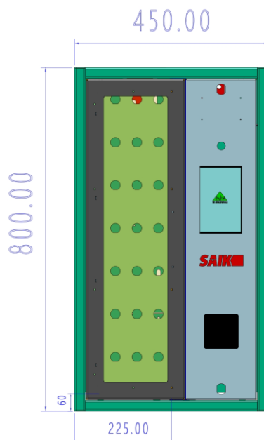
rysunek techniczny [schematic drawing]
