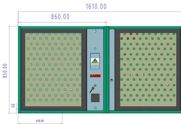
rysunek techniczny [schematic drawing]
