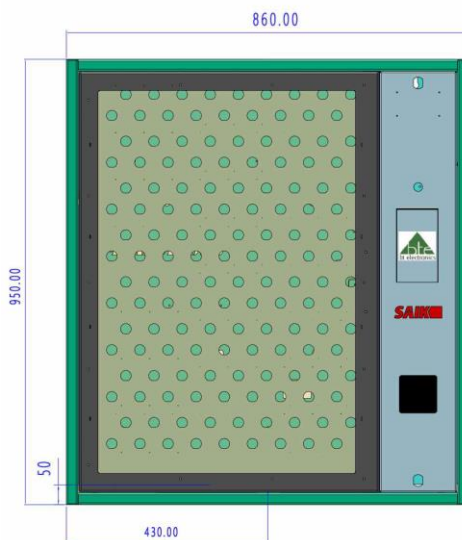
rysunek techniczny [schematic drawing]
