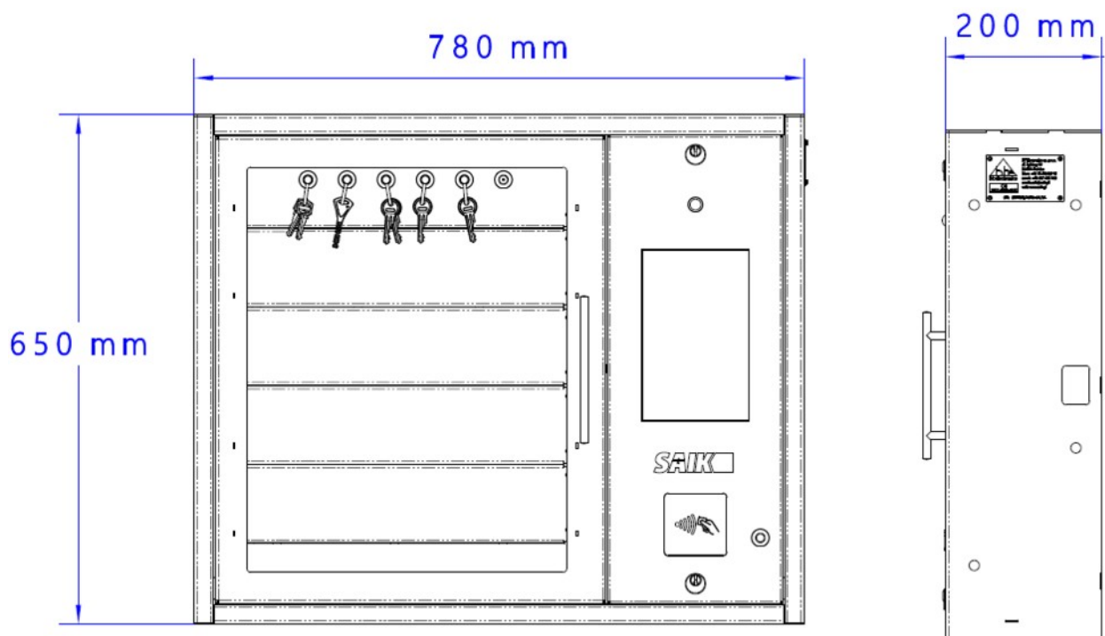
Rysunek 1 SAIK MODULE 60 rysunek techniczny
