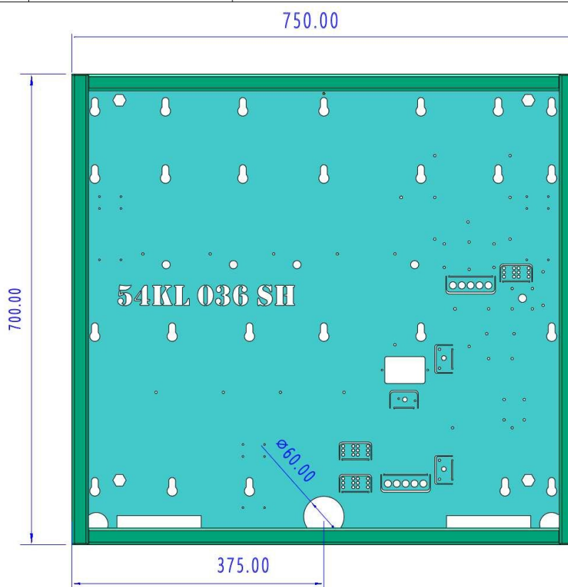
Przykładowe zdjęcie tyłu depozytora z zaznaczonym otworem do okablowania
